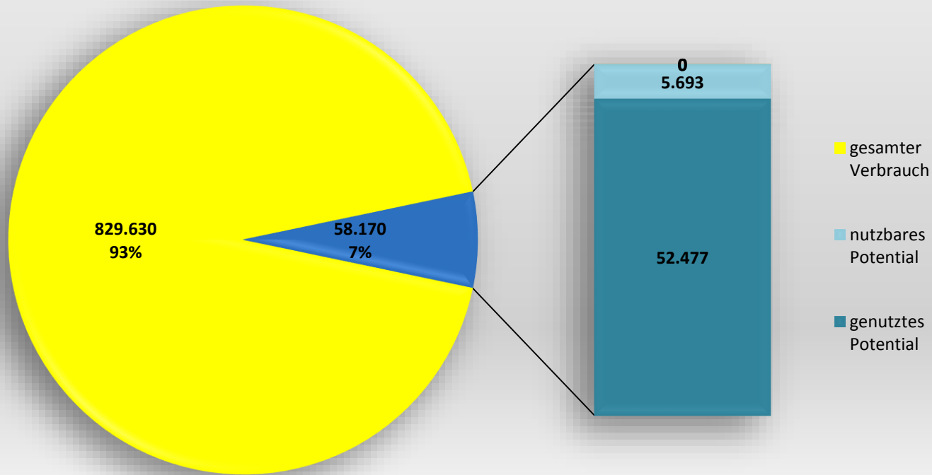
Stromverbrauch und Deckung LKR Passau in MWh/a
